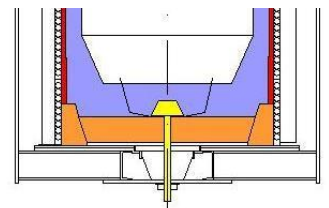
Tapón Poroso
