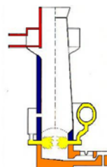
Cubilote
